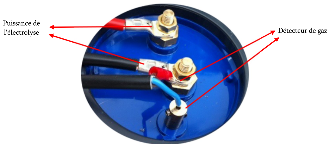
Fig 5 – Bornes de connexion de cellule d'électrolyse
